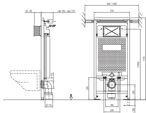
Instalační splachovací modul G se vzpěrou
