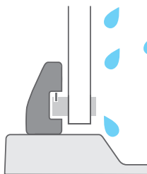
Rám ve spodní části koutu: 10°, Pivot, Blix Slim, Blix, Supernova
