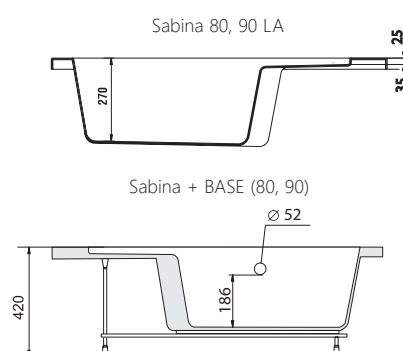
TYP LA + BASE + SET vanička LA s nožičkami a panelem
