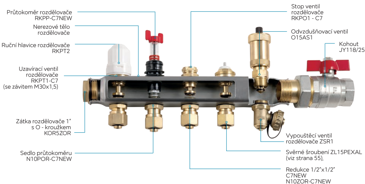
Profil NEREZ
