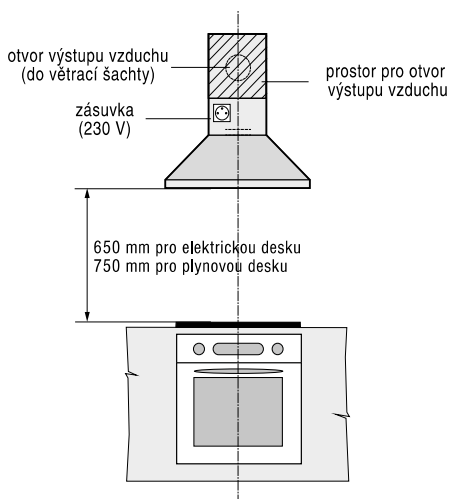
Základní umístění komínového odsavače nad pracovní varnou deskou
