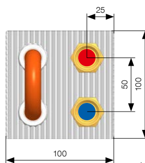
typ 22
