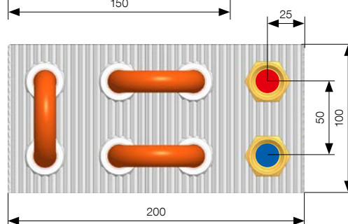
typ 42
