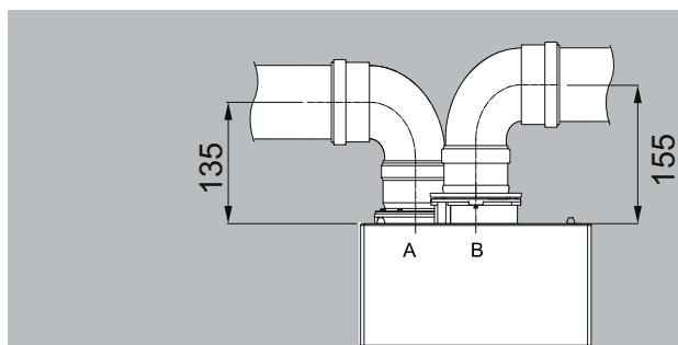
Dělené odkouření Ø 80/80
