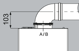
Koncentrické odkouření Ø 60/100
