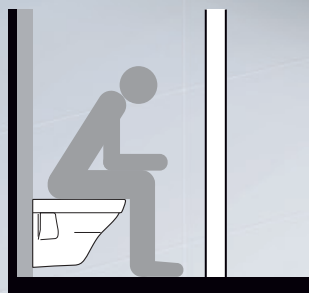
závesný klozet 49 cm a podomítkový modul 8 cm závesný klozet 49 cm a podomietkový modul 8 cm
